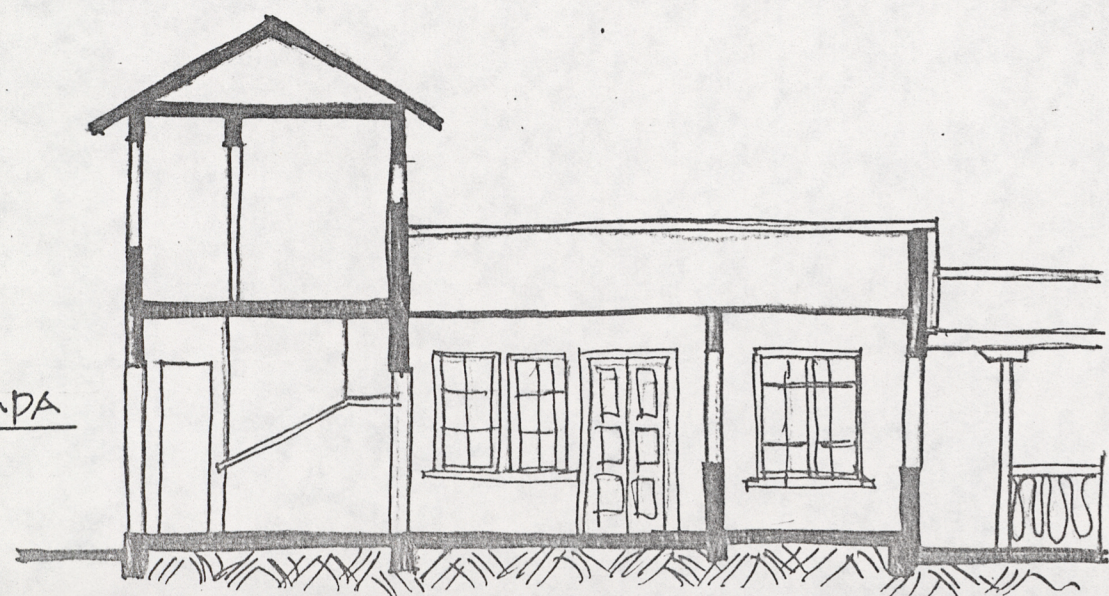
CASA COMPLETA
