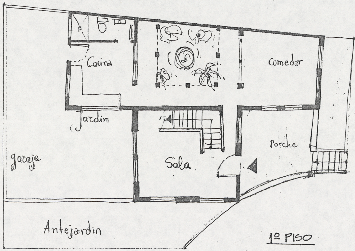
PLANO ESCALA: 1:100
