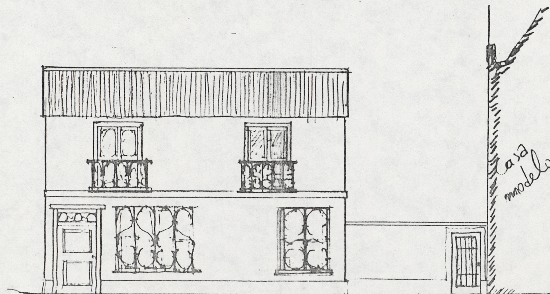
FACHADA
