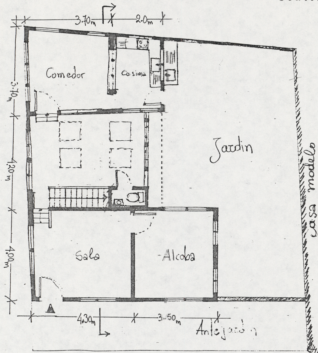
PLANO ESCALA: 1:100 1º PISO
