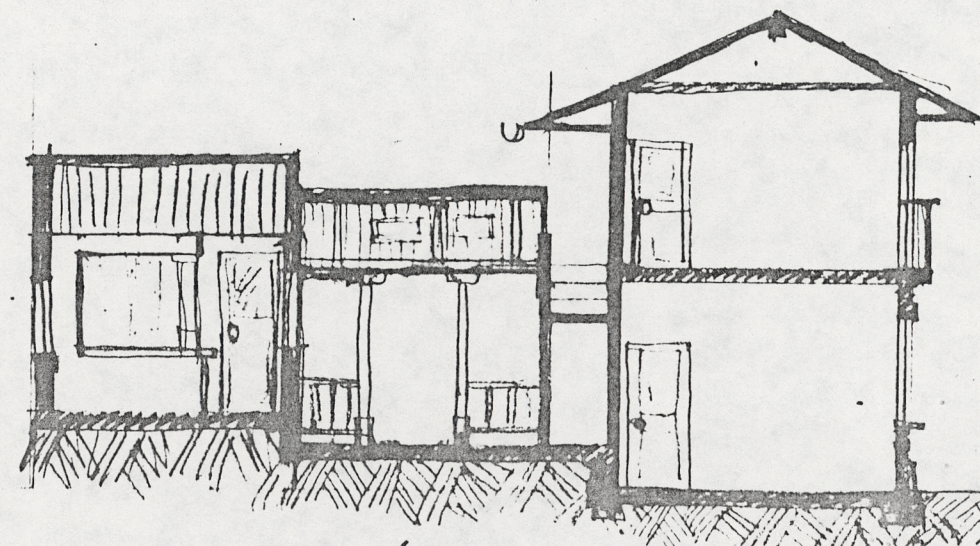
SECCIÓN
