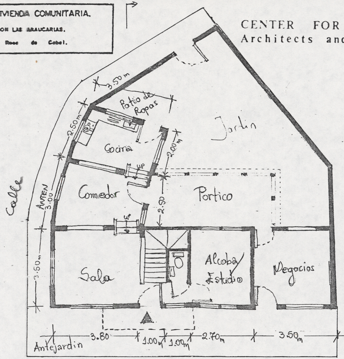
1º PISO Calle PLANO ESCALA - 1:100
