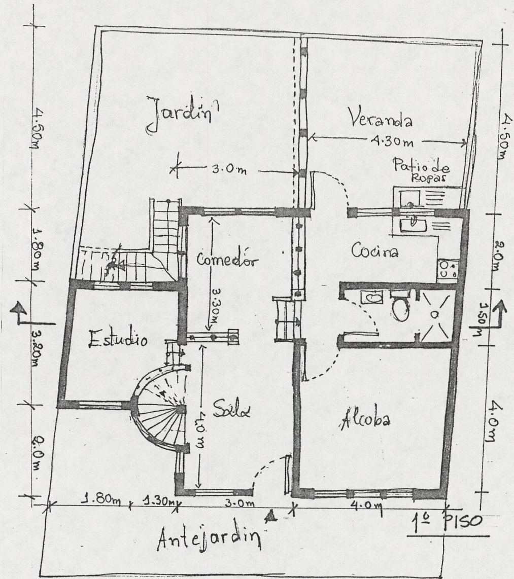
PLANO ESCALA: 1:100
