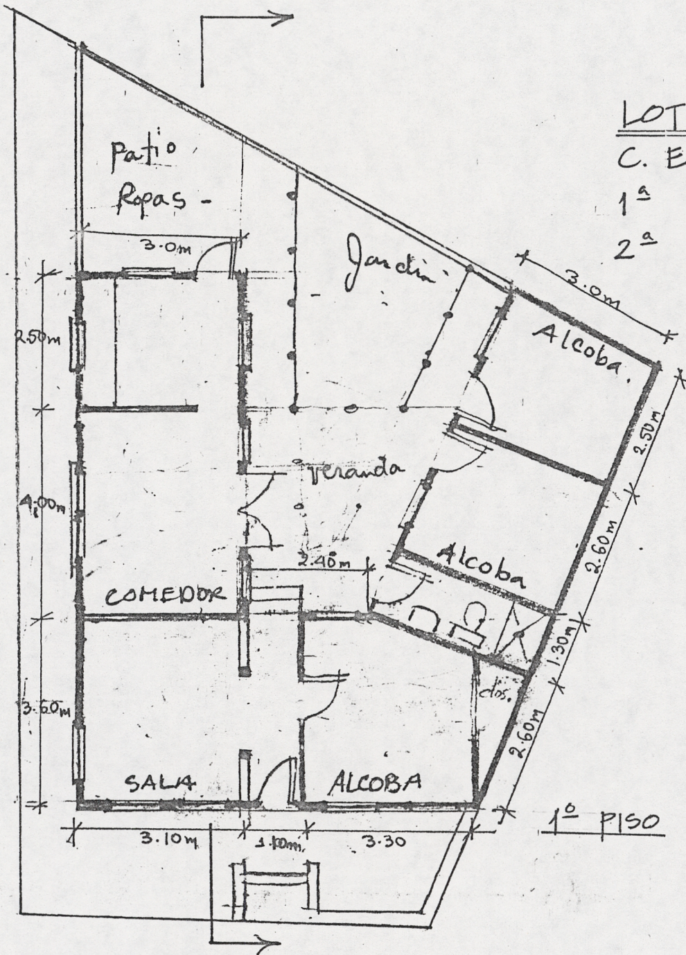
PLANO ESCALA - 1:100
