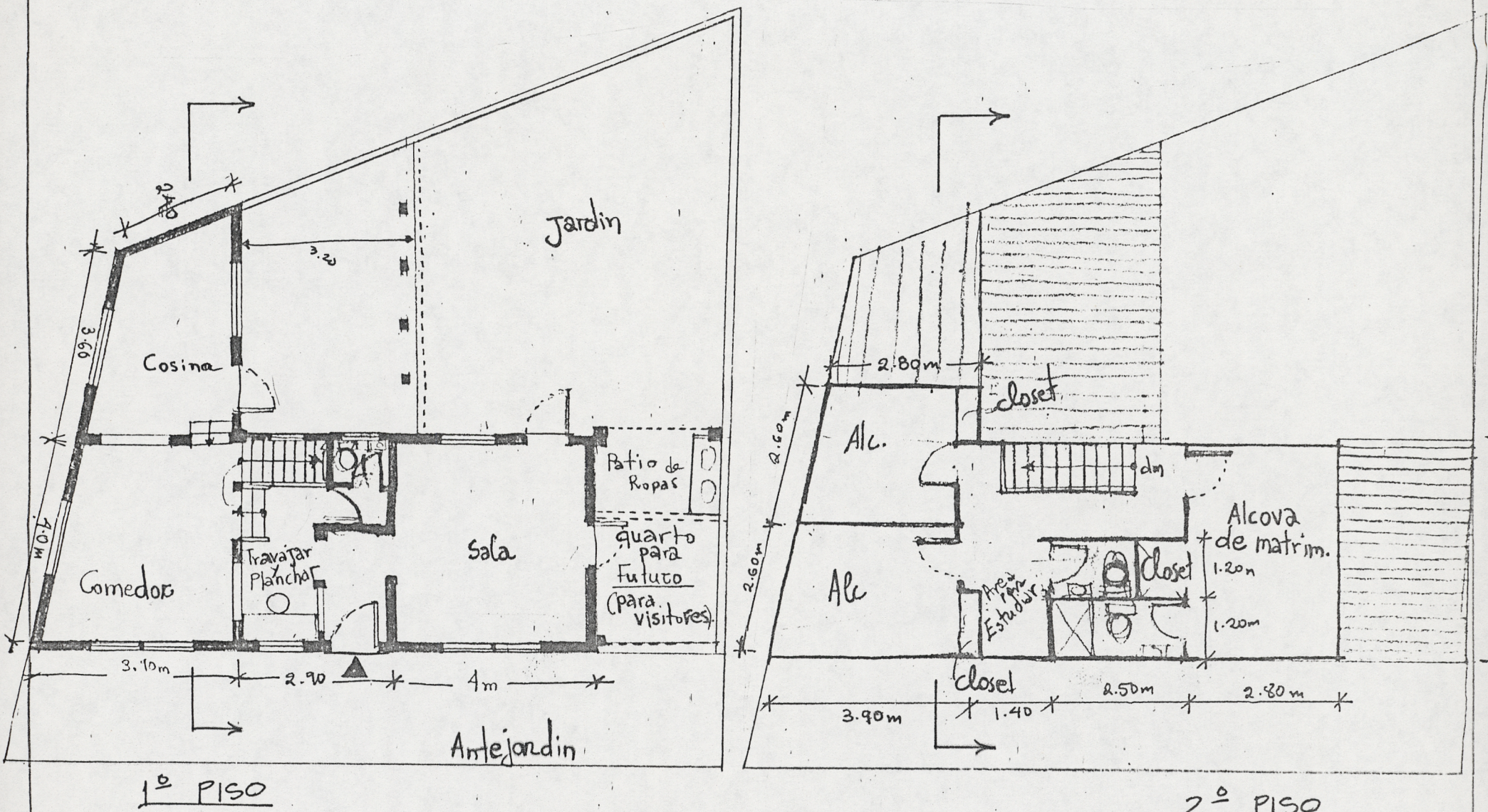
PLANO ESCALA - 1:100
