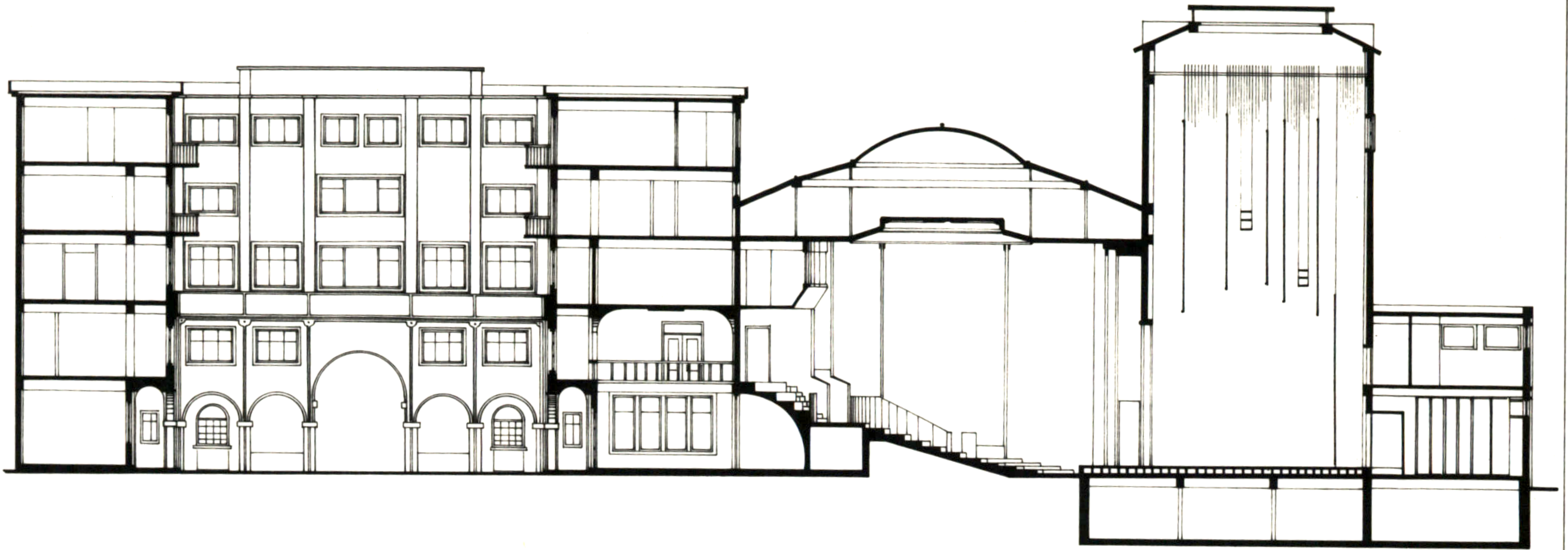
SECTION a-a
