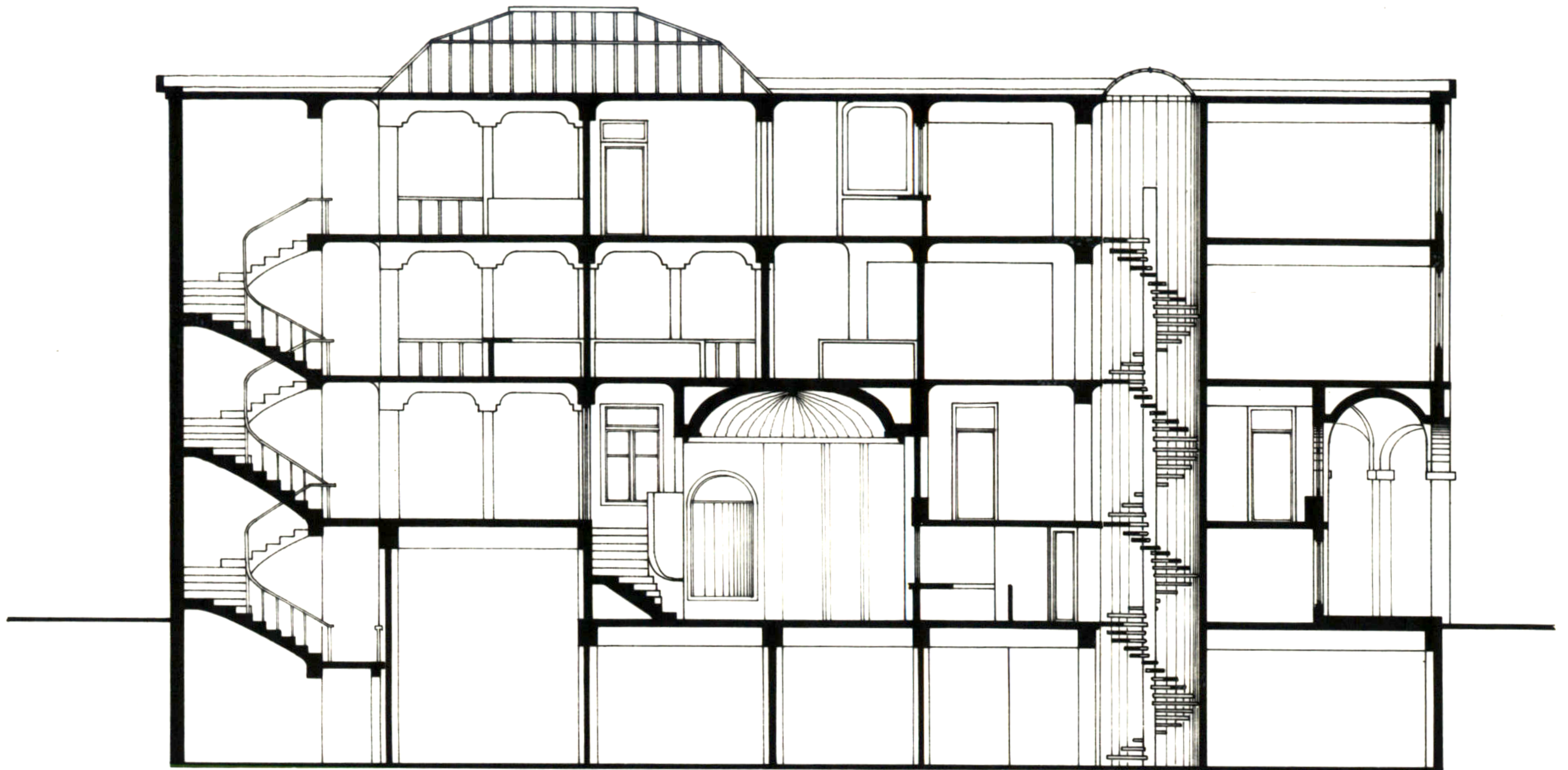
SECTION a-a
