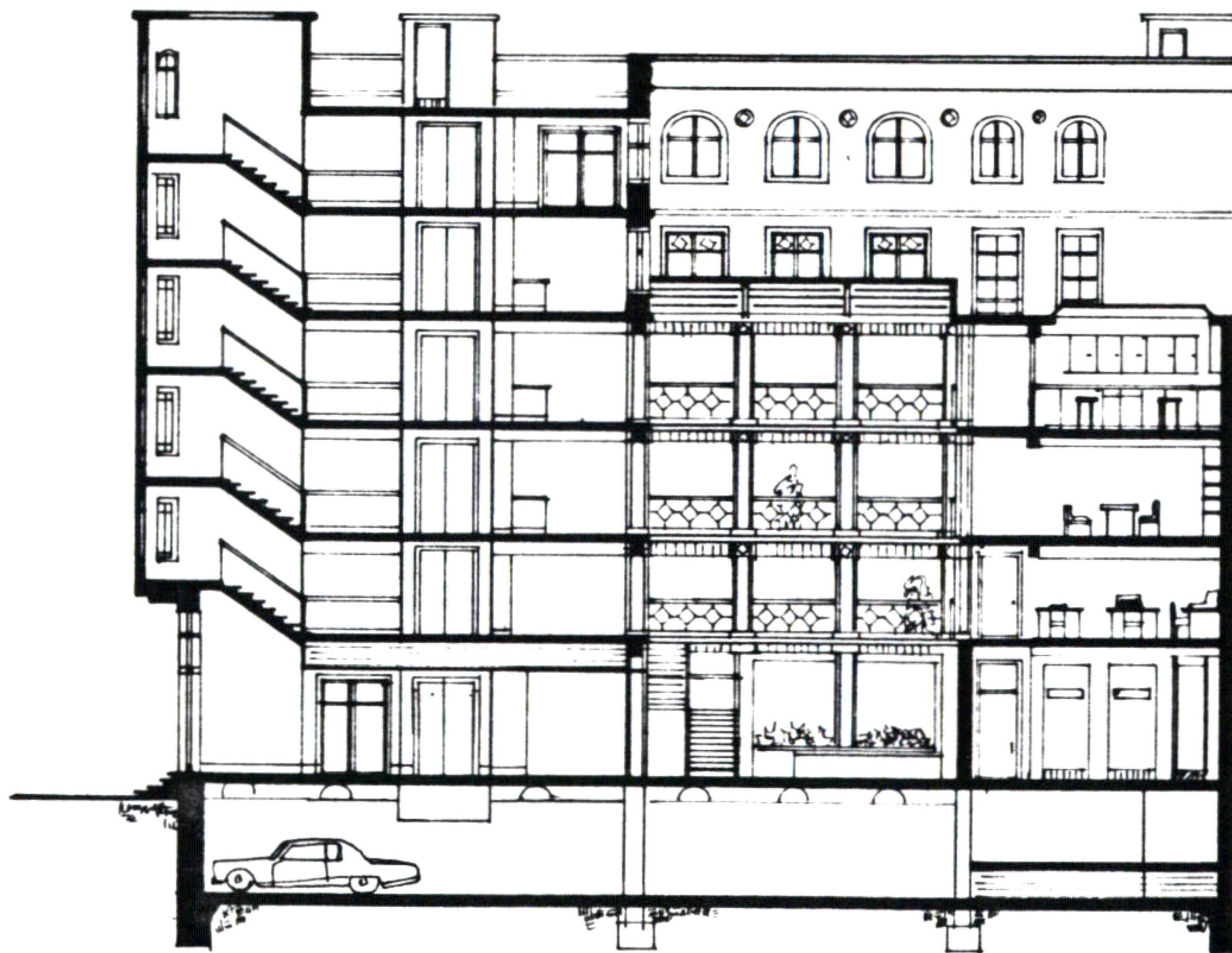
SECTION A-A
