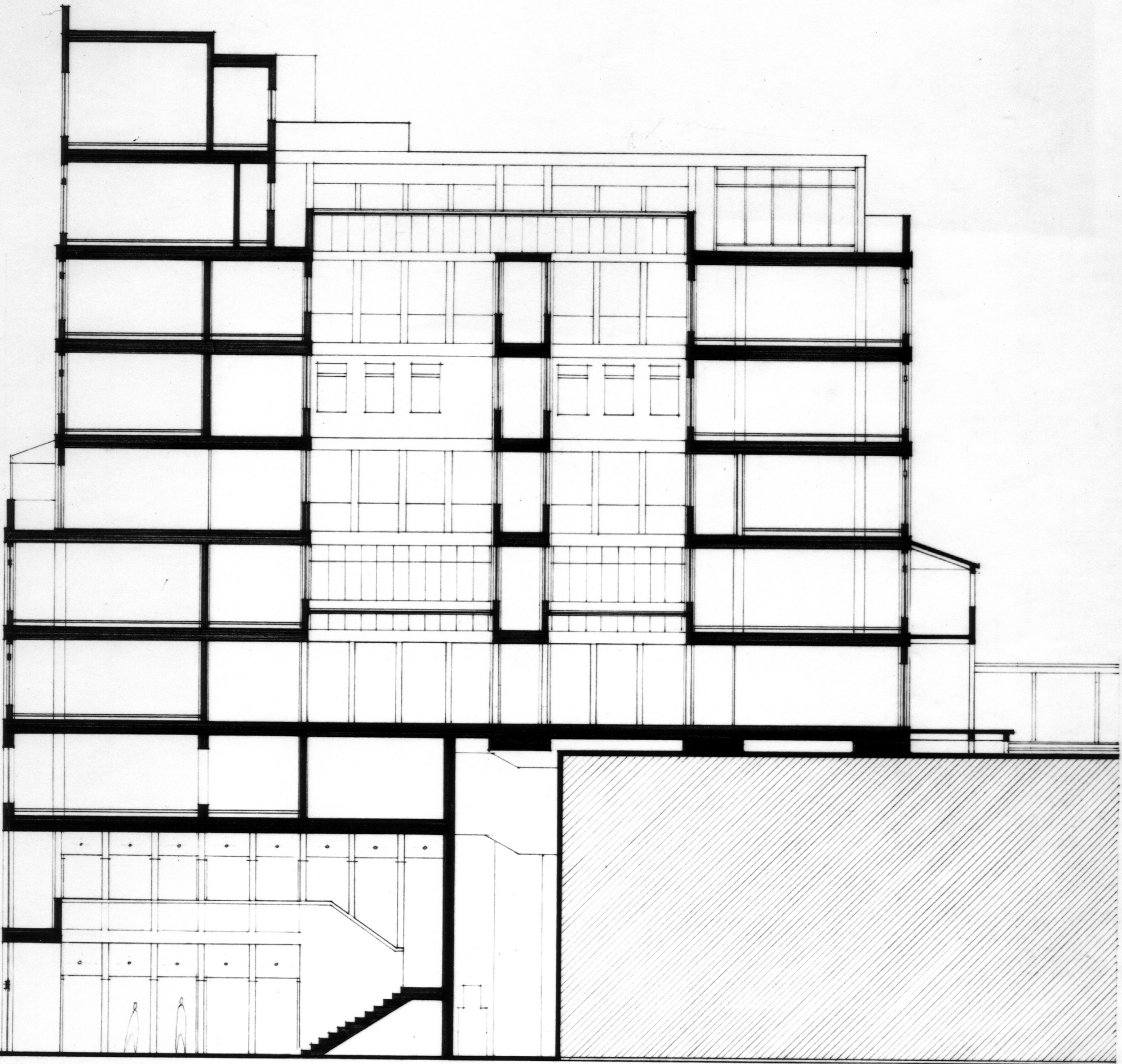
longitudinal section
