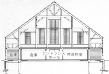
断面 section
