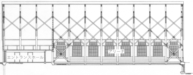
断面 section S=1:500
