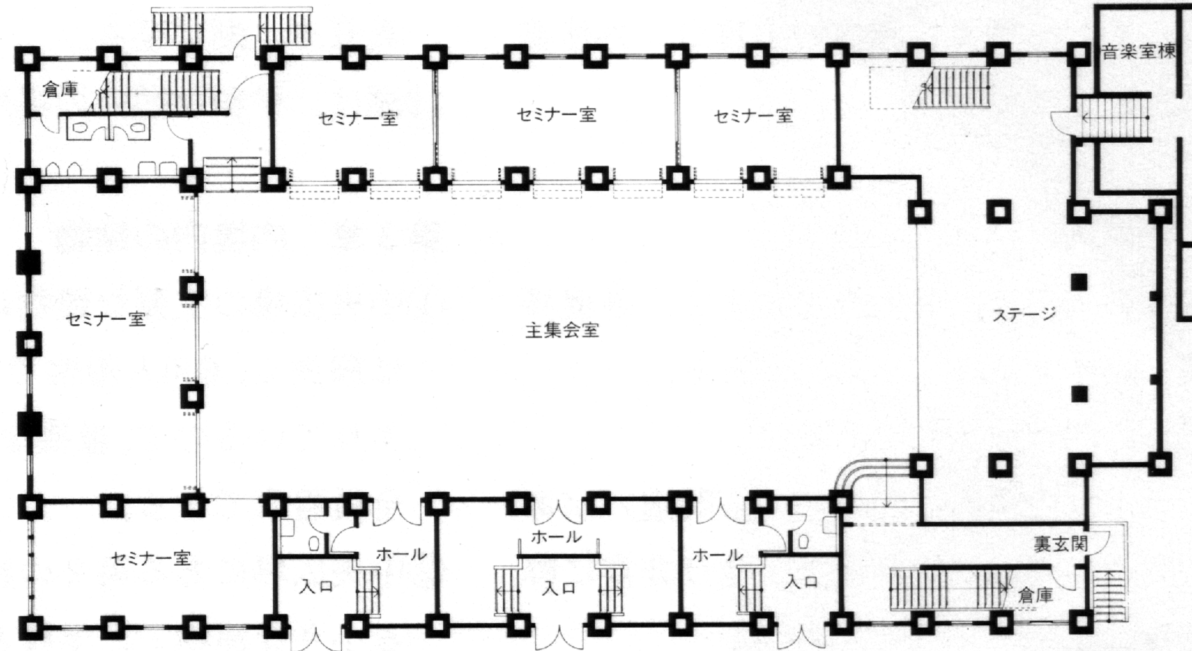
大講堂 1階平面 縮尺 1/500
