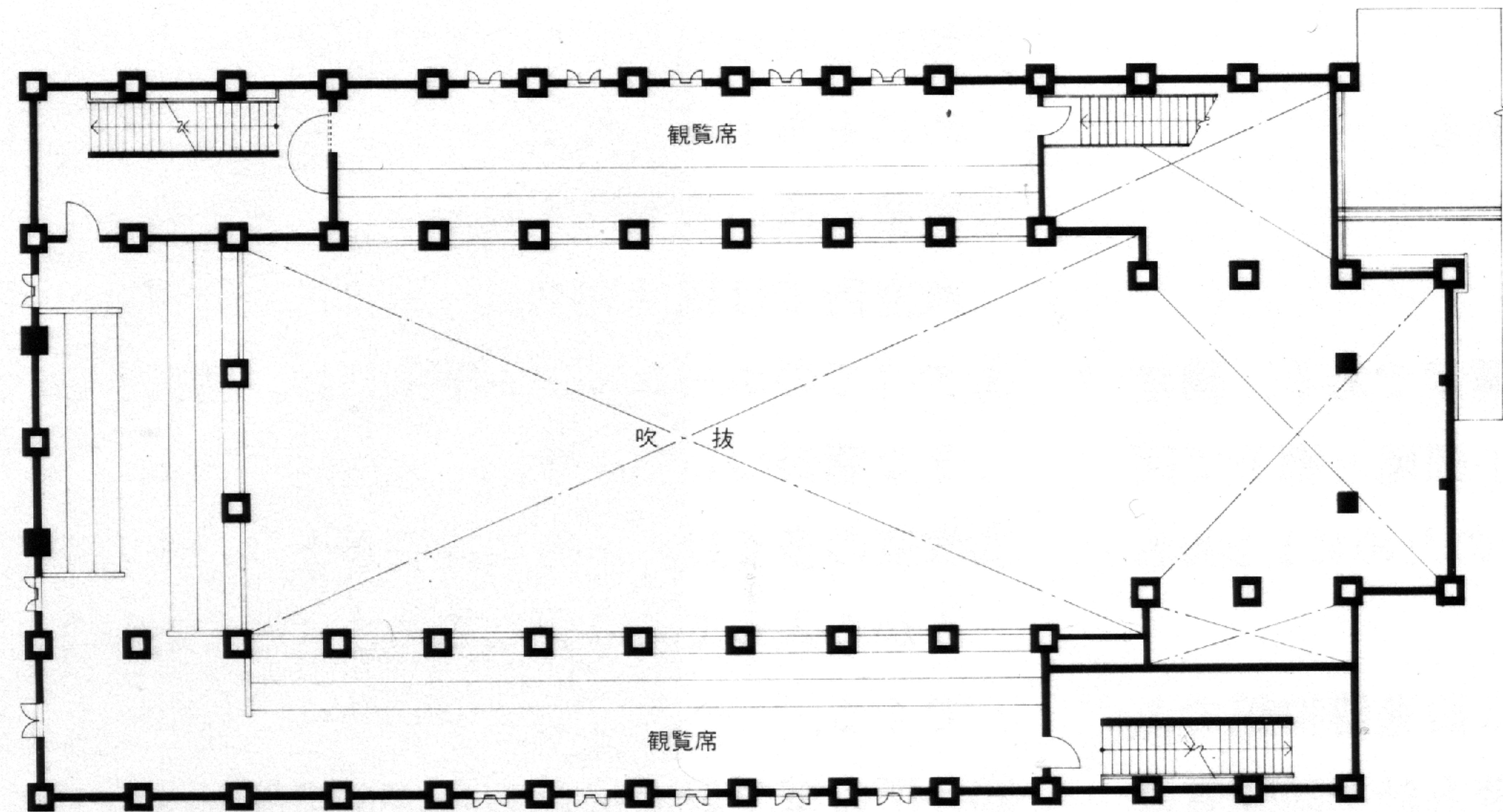
大講堂 2階平面
