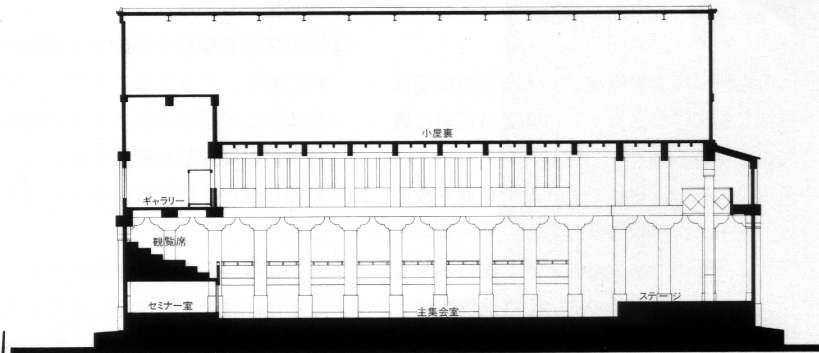
大講堂断面 縮尺 1/500
