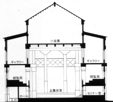
大講堂断面
